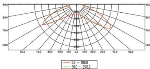
T-I (120°)
