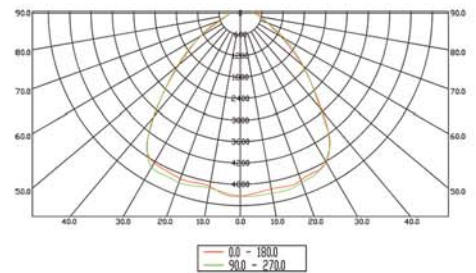
T-V (90°)
