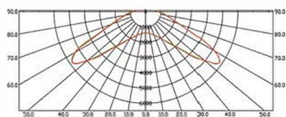
T I-1 (120°)
