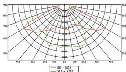
TI-2 (80° * 136°)
